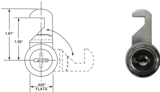
3500-100 (Door)
