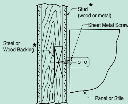
Stud Wall
