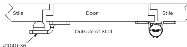
Fig. 11d: Perpendicular/Inswing Door
