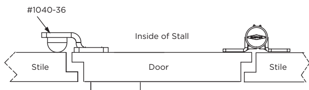
Fig. 11b: Inswing Door
